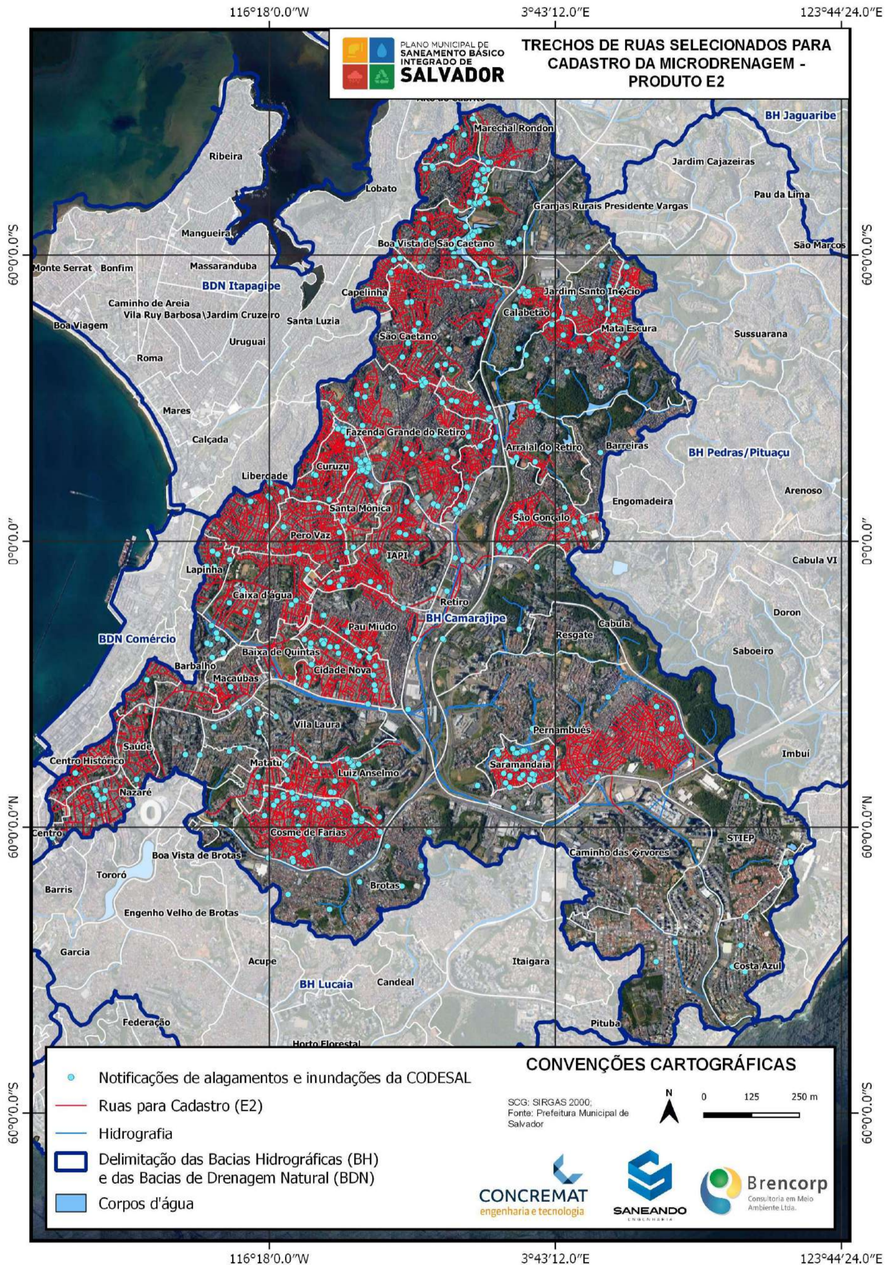
Figura 4 – Trechos de ruas selecionados para cadastro de microdrenagem – Produto E2
