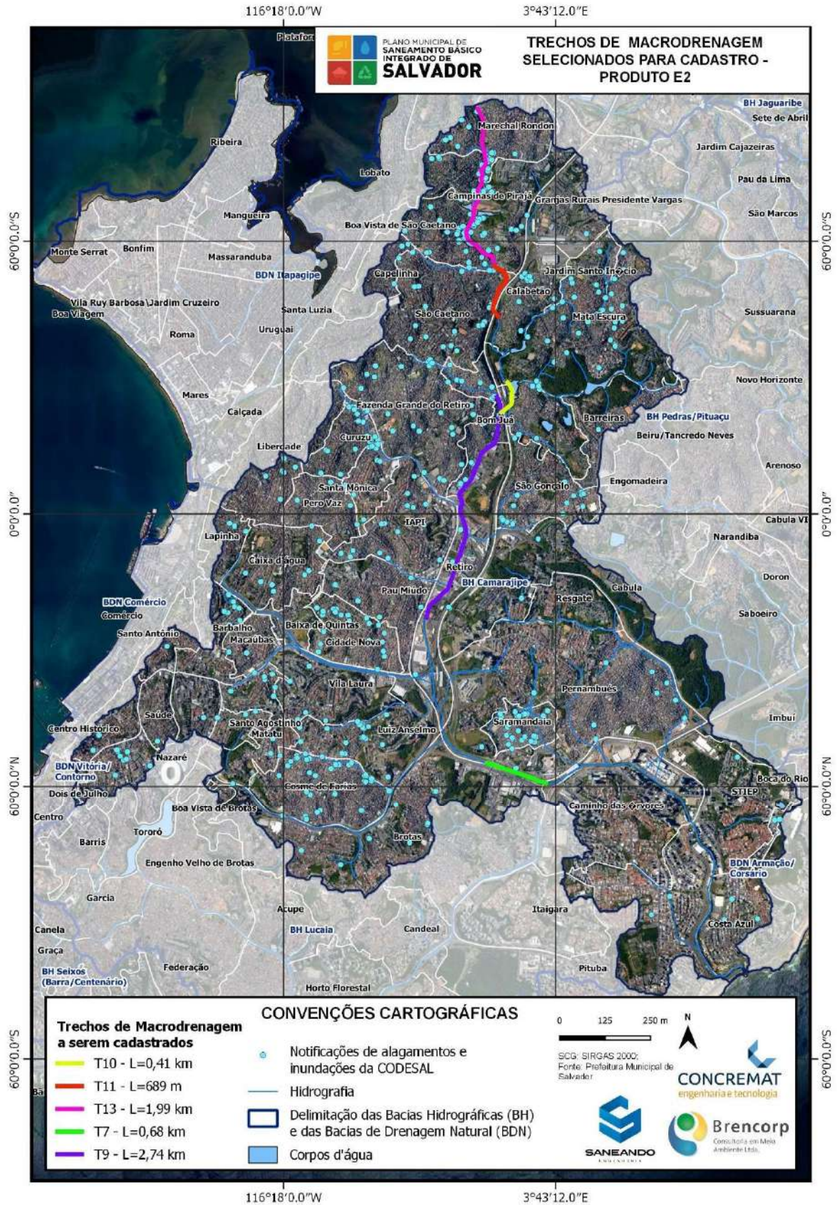
Figura 6 – Trechos de macrodrenagem definidos para o Produto E2
